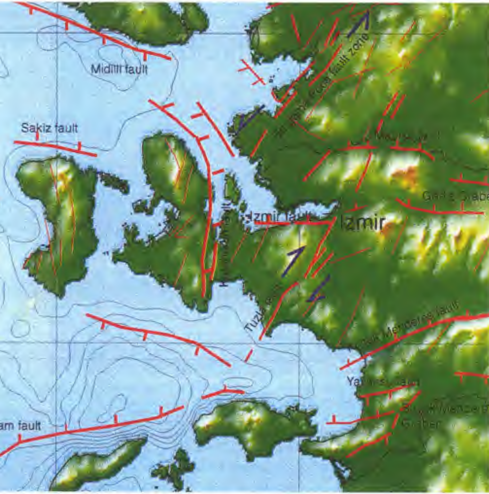
Izmir ve çevresi fay haritası
